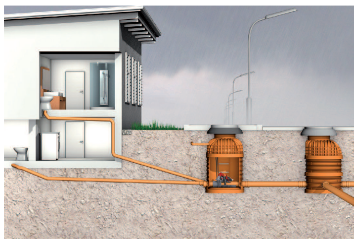
Žádné vzduť odpadní vody ve sklepě díky zabezpečení proti vzduť REHAU „Quatrix-K“ pro odpadní vody s obsahem fekálií
